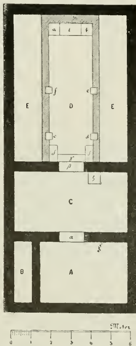
93. sz. Az aquineumi Mithraeum alaprajza; A) előcsarnok, B) ismeretlen rendeltetésű e'zart fulke alpha) bejárat a vestibulumba, C) vestibulum (pronosz), gamma) szobortalapat, beta) gamma) a cellál az vezető bejárat lépcsői, D) szentély (cella), E) oldal folyosók, delta) feljárat az oldal folyosókhoz, alpha) Mithras petrogenitus (sziklából született) szobra, epsilon) Mithras-tábla helye, l) egy másik szobor talapzata, c, d) e) f) fogadalmi oltárok. Kuzsinszky Bálint dr. után. Arch. Ért. u. f. VIII. köt. 287. l. után.
